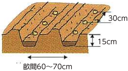
図1 畑の準備
