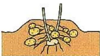
図5 収穫
